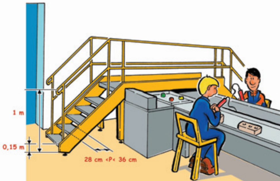
Passerella con parapetto, sopra una linea di produzione
