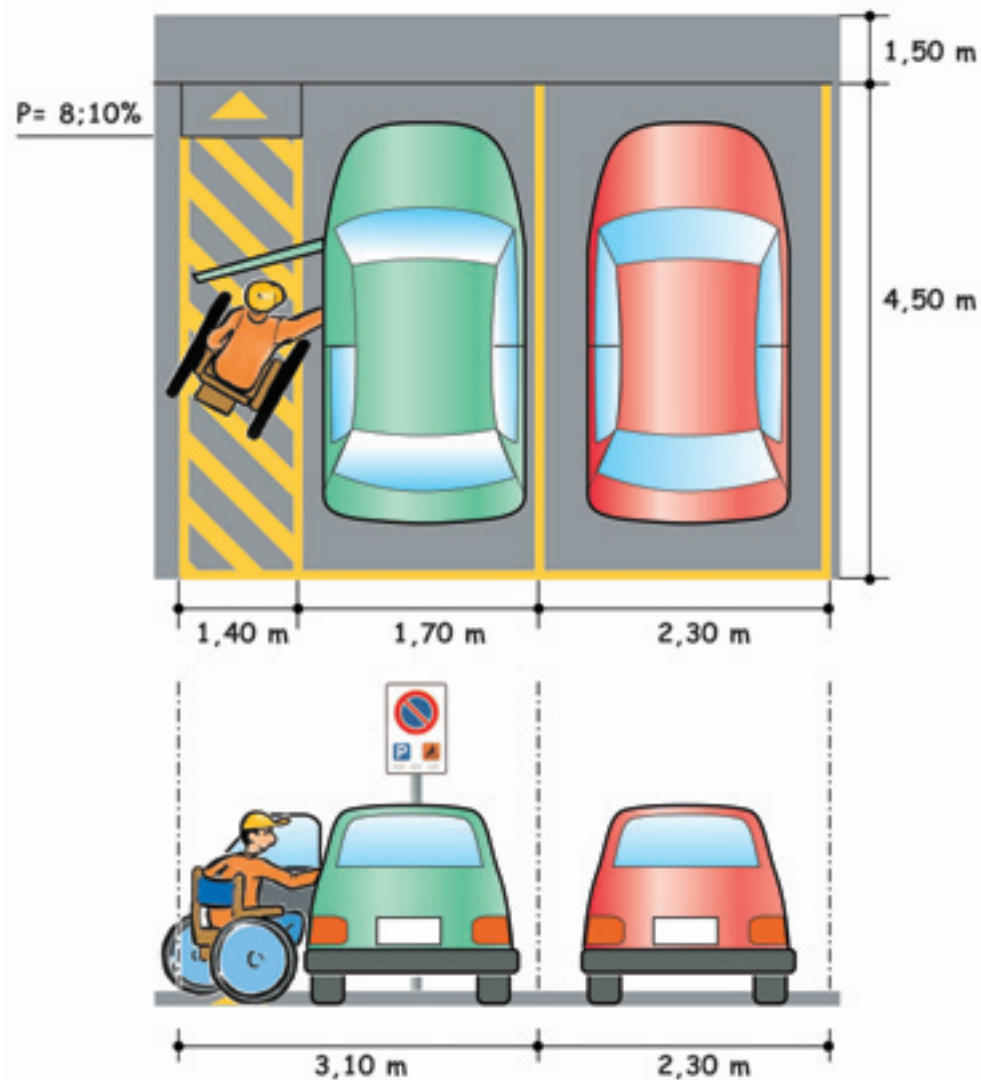
Caratteristiche e dimensioni minime di uno stallone di sosta riservato alle autovetture per i disabili
