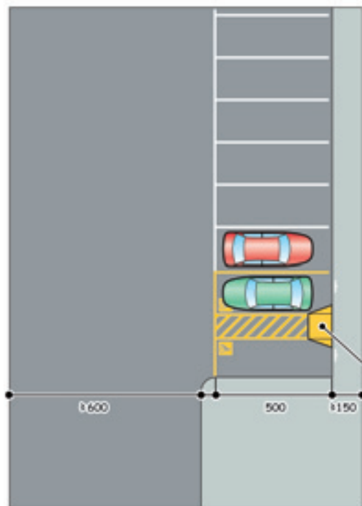
Schema indicativo di un impianto di parcheggio "a pettine" per autovetture con 2 posti auto, abbinati per le persone disabili
