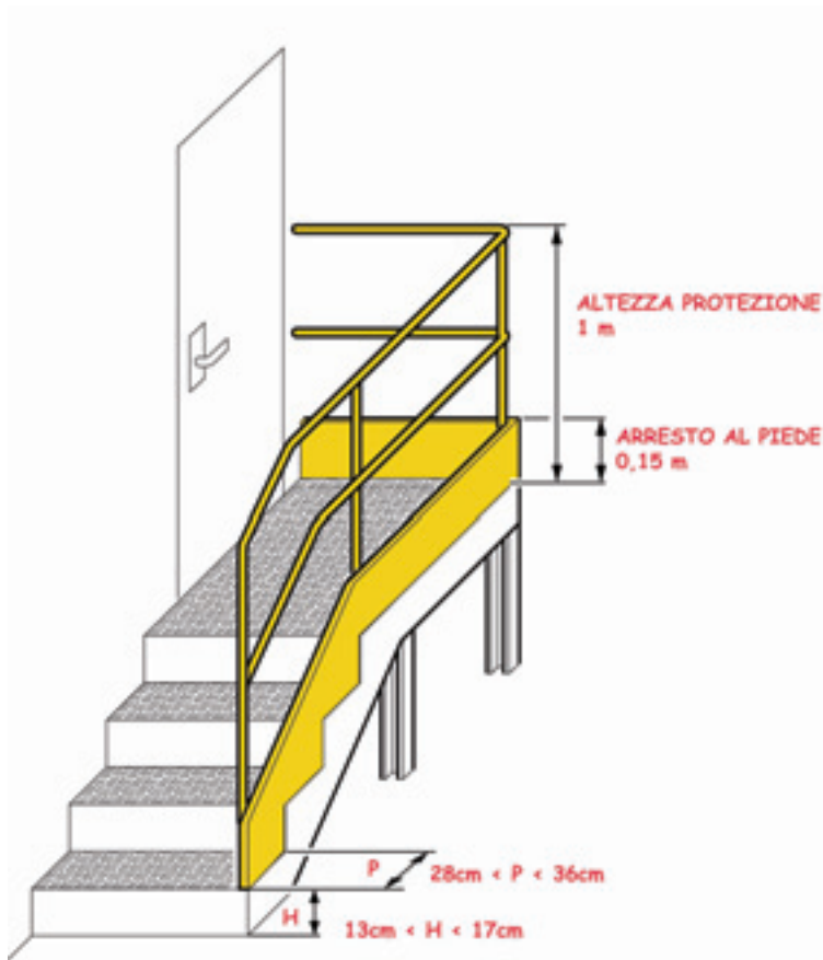
Dimensioni degli elementi costitutivi di una scala
