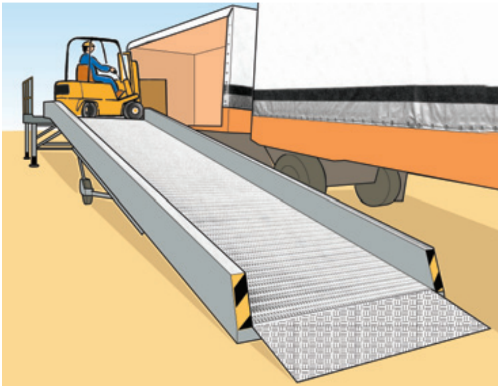
Rampa di carico mobile, dotata alla sommità di piattaforma di manovra, utilizzata per le operazioni di trasbordo dei mezzi a partire dal livello del suolo
